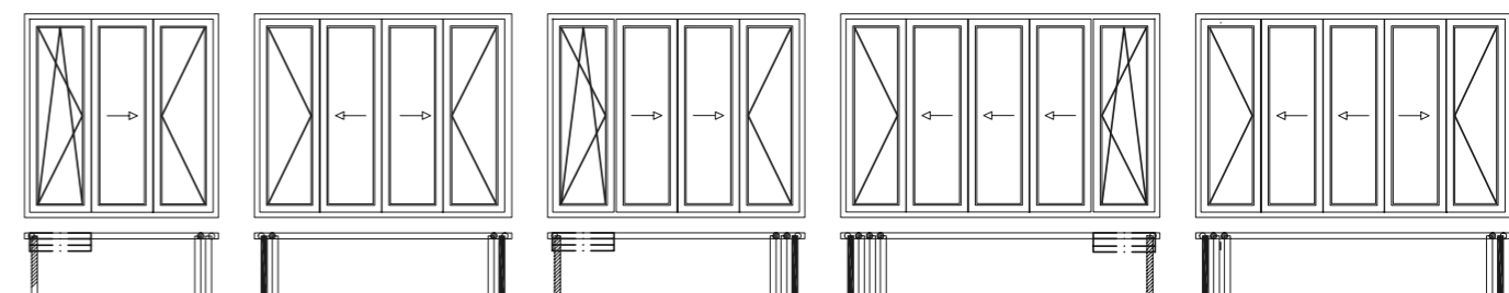
Sheme - mogućnosti otvaranja sustava PremiFold 76
