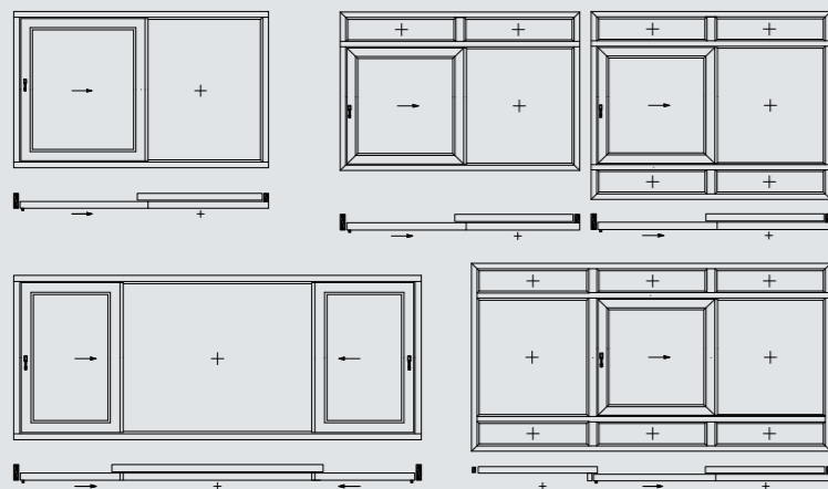
Scheme otvaranja kliznih stijena Premislide 76
