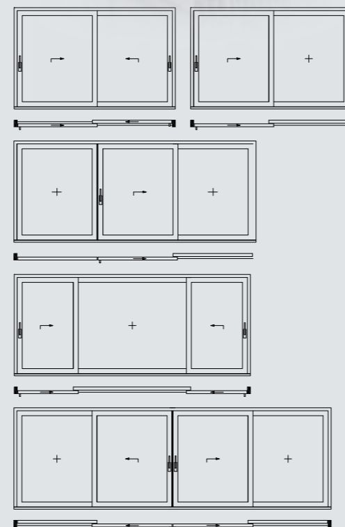
Sheme otvaranja kliznih stijena PremiDoor 76 i PremiDoor 88
